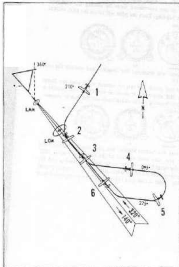
ILS FRONT COURSE APPROACH
