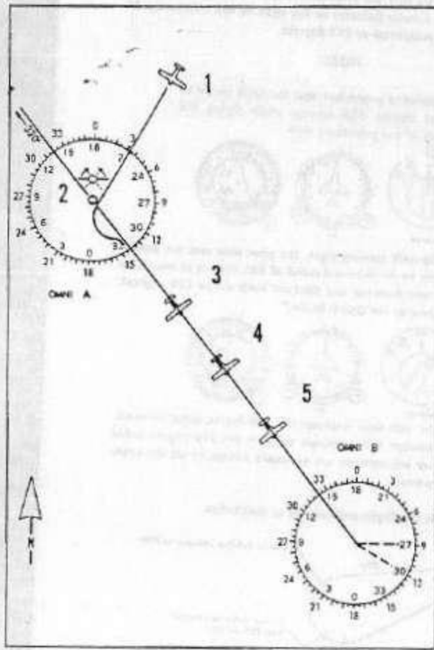
VOR NAVIGATION
