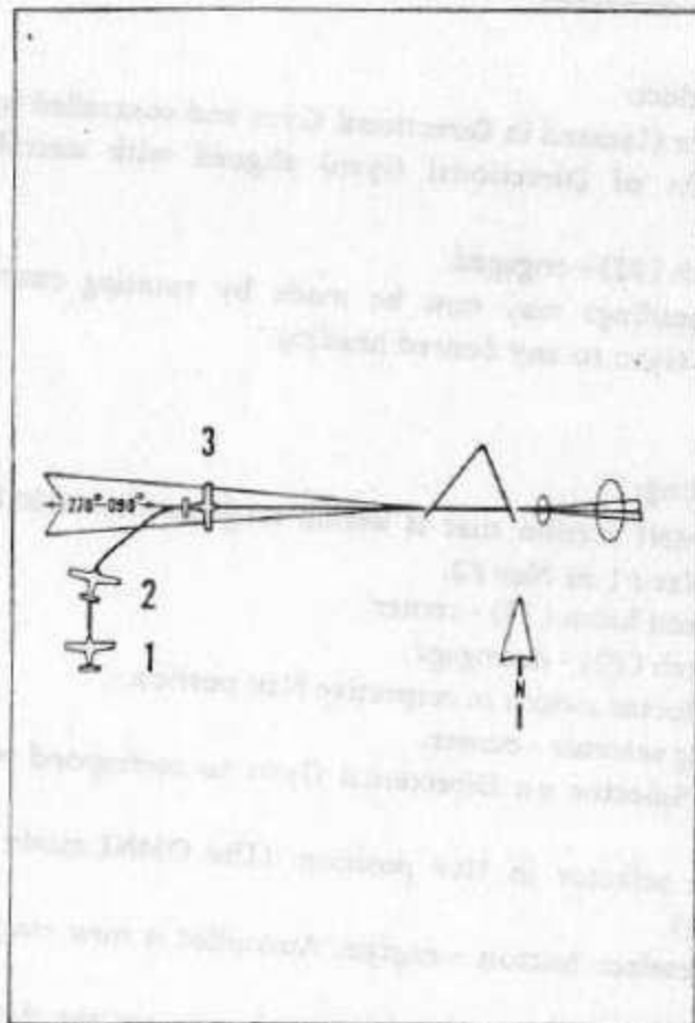
ILS BACK COURSE APPROACH
